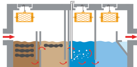
嫌気ろ床槽 ばっ気槽 沈殿槽
